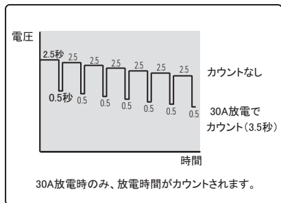
パルス放電のカウント例
